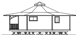
4 REAR ELEVATION Scale: 1/8" = 1'-0"
