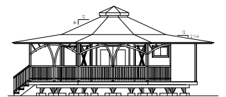
3 SIDE ELEVATION Scale: 1/8" = 1'-0"
