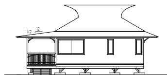
5 SIDE ELEVATION Scale: 1/8" = 1'-0"
