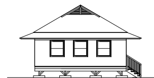
6 REAR ELEVATION Scale: 1/8" = 1'-0"
